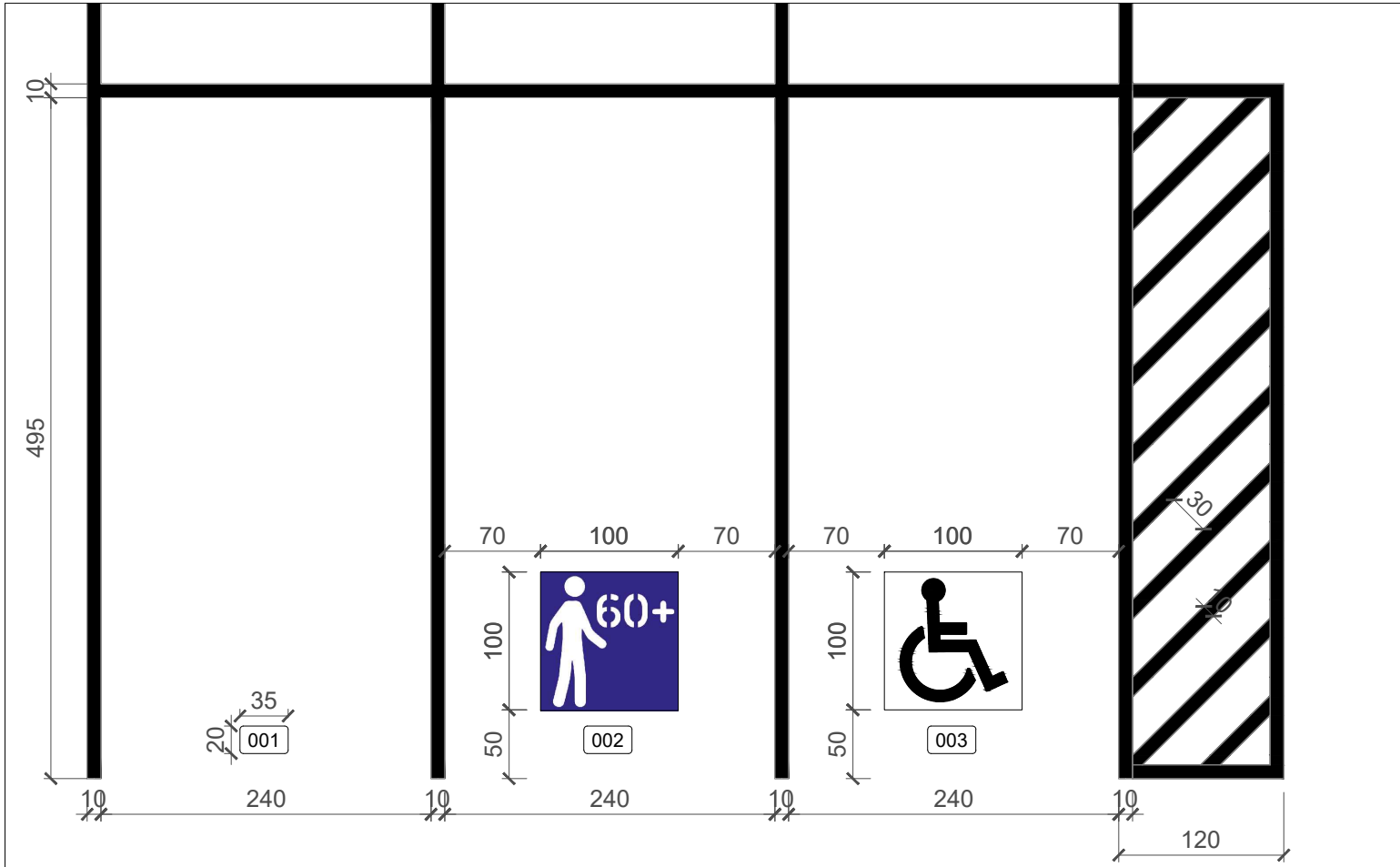
Detalhe de sinalização horizontal para as vagas de estacionamento
