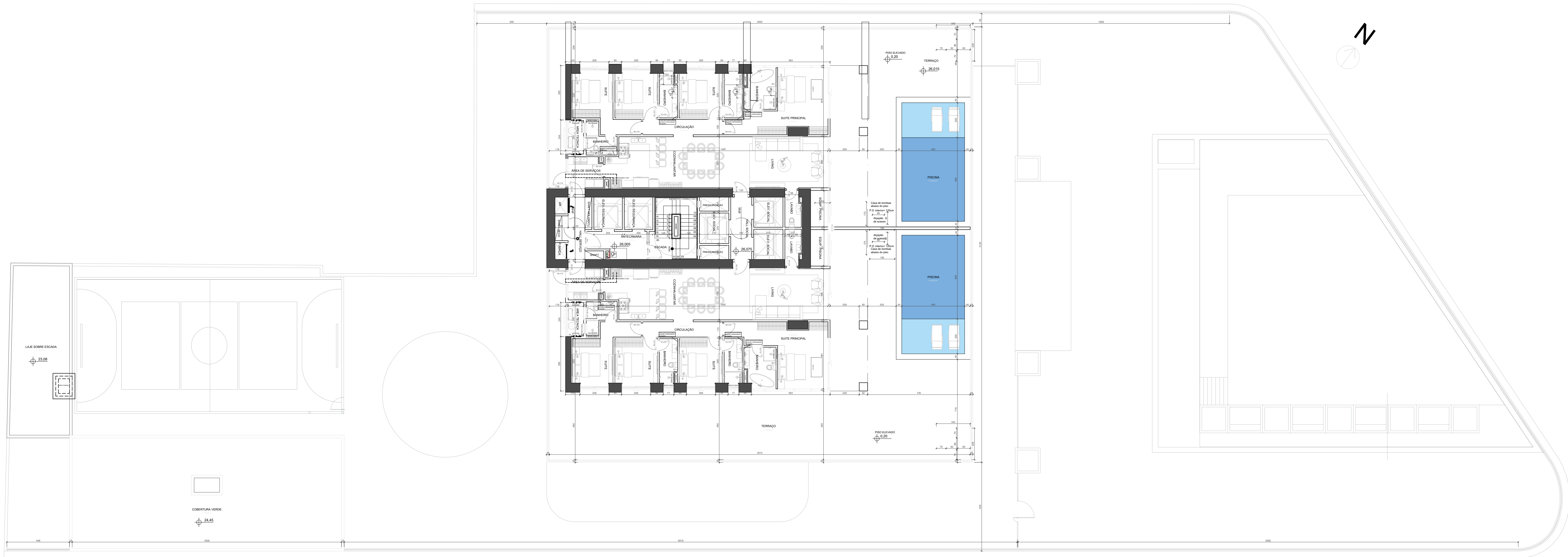
PLANTA BAIXA - PAVTO TIPO DIF. 01 ÁREA DO PAVTO= 922,43 m² ÁREA PRIVATIVA= 394,36 m² ÁREA PRIVATIVA= 485,88 m²
