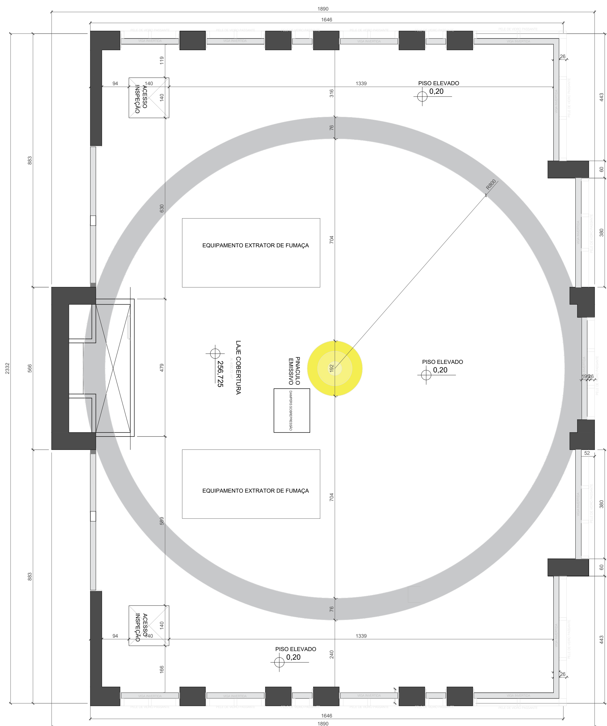
PLANTA BAIXA - LAJE COBERTURA ÁREA DO PAVTO= 400,72 m²
