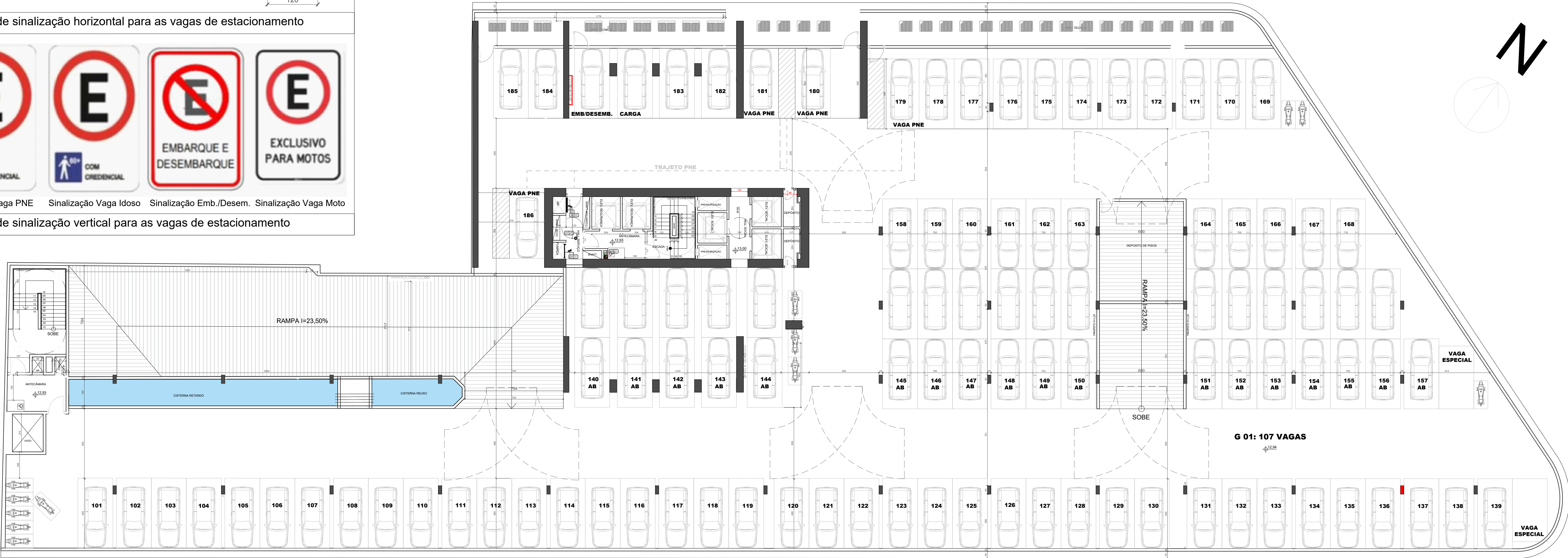
PLANTA BAIXA - GARAGEM 01
