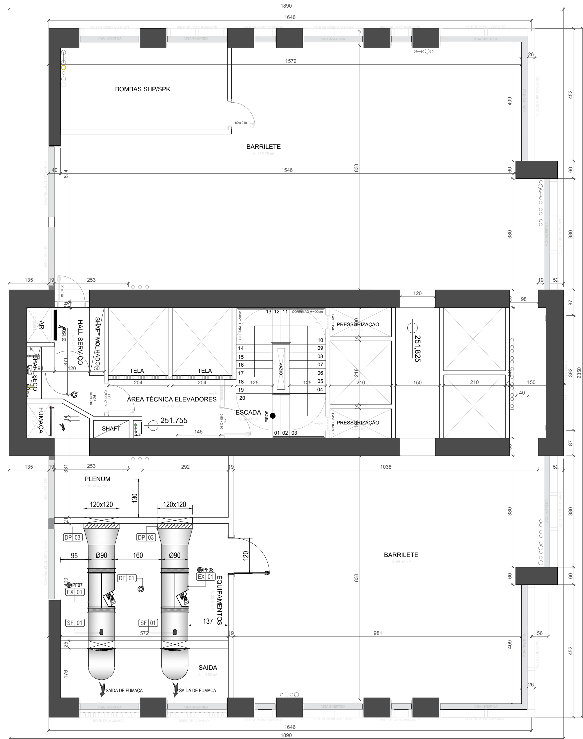
PLANTA BAIXA - BARRILETE ÁREA DO PAVTO= 372,27 m²
