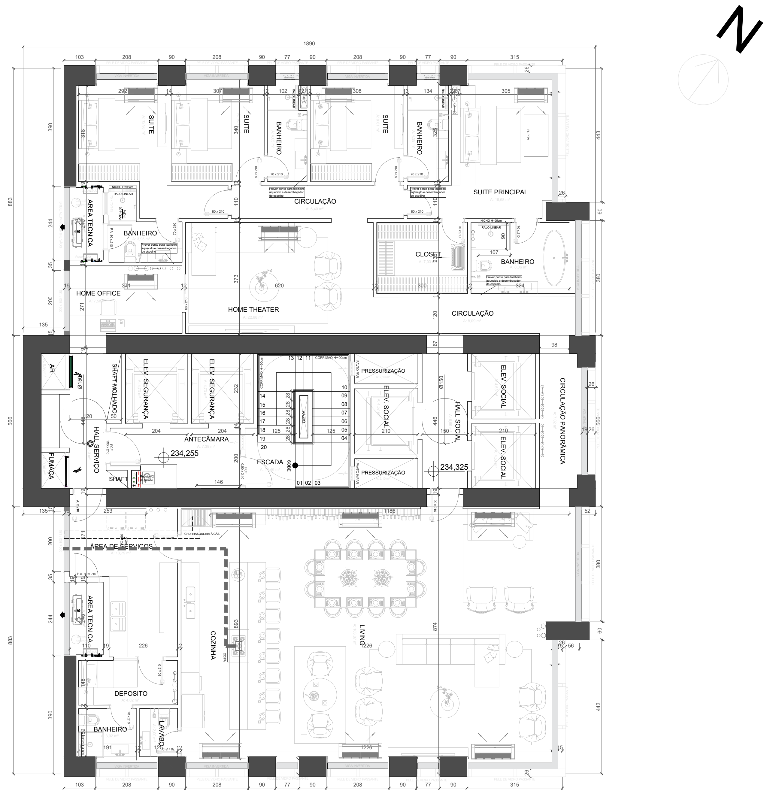
PLANTA BAIXA - PAVTO TIPO MASTER ÁREA DO PAVTO= 372,27 m² ÁREA PRIVATIVA= 307,96 m²
