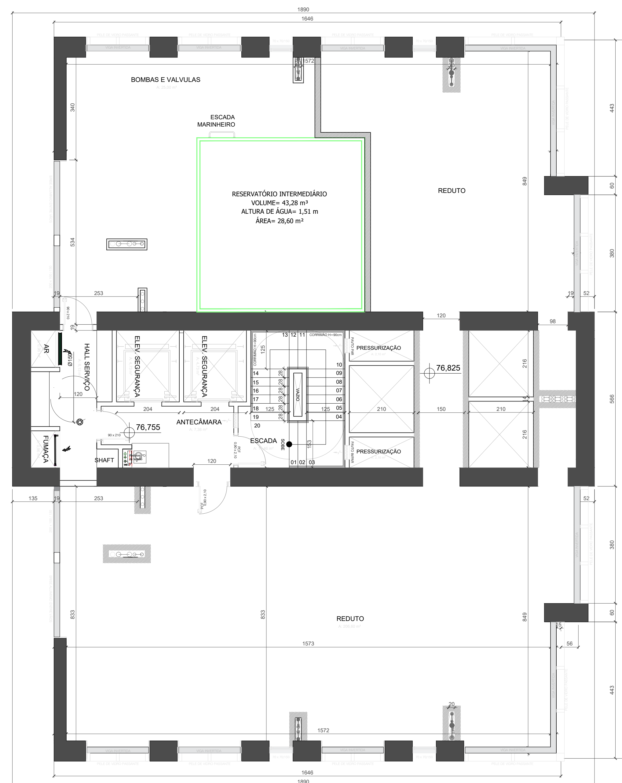
PLANTA BAIXA - PAV. TÉCNICO ÁREA DO PAVTO= 372,27 m²
