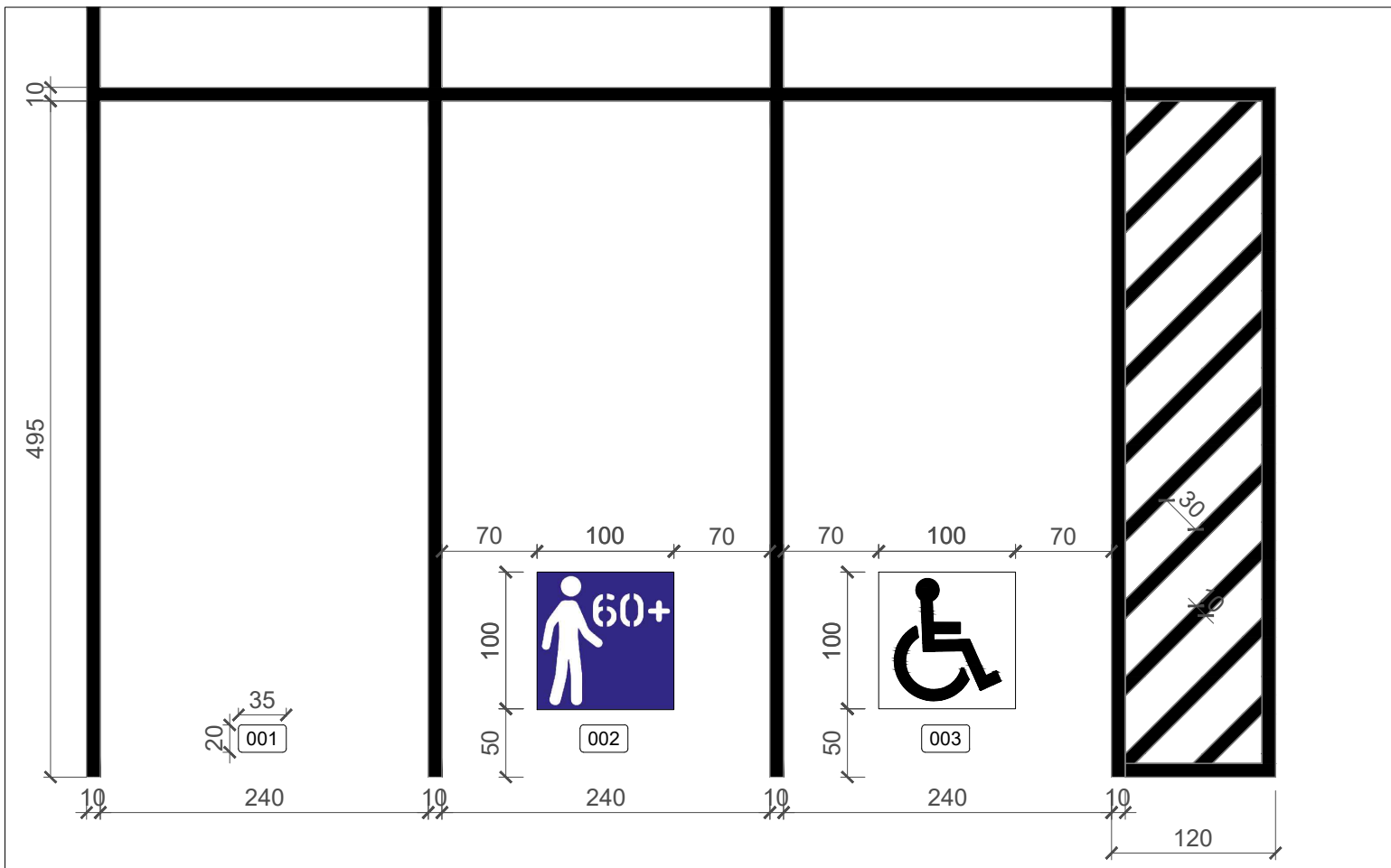
Detalhe de sinalização horizontal para as vagas de estacionamento
