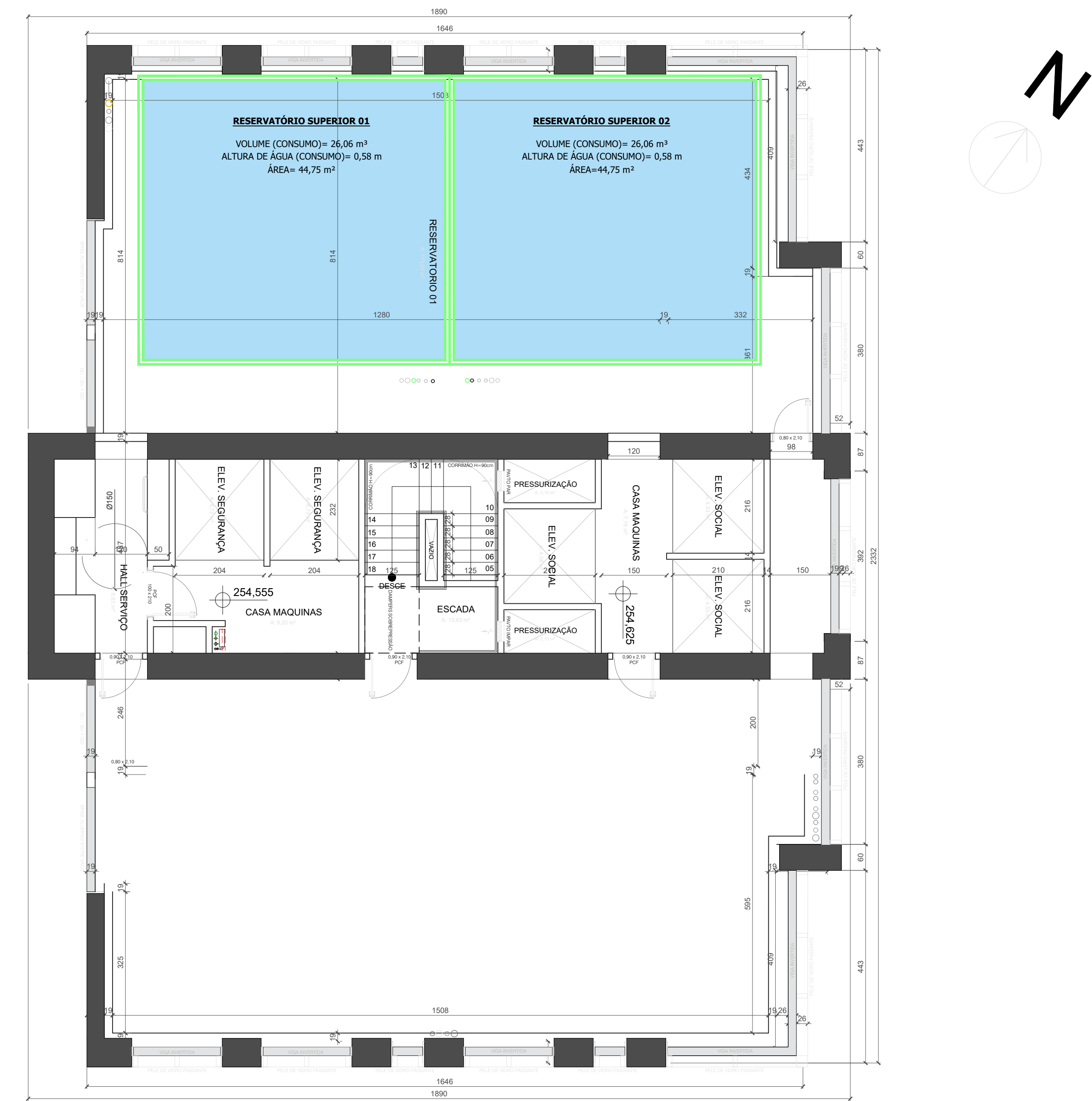
PLANTA BAIXA - CASA MAQUINAS E RESERVATORIOS ÁREA DO PAVTO= 372,27 m²
